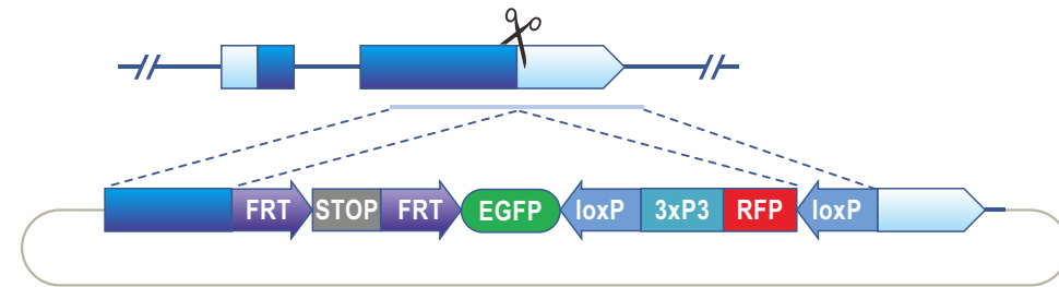
dsDNA Donor
